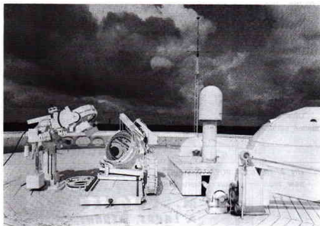
— Ce que l'on peut voir sur la plate-forme de la tour solaire : le créostat à deux miroirs a été découvert, la coupole (en partie visible à droite du cliché) ayant été soulevée puis déposée automatiquement; entre le créostat et la coupole, on distingue le support qui était destiné à l'instrument d'observation des satellites.
